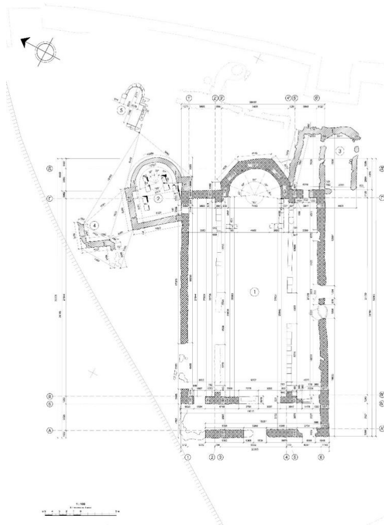
Рис. 10. План Западной базилики Херсонеса (план Е.В. Огиенко) (Фомин М. В., Огиенко Е. В., Шевцова А. А. 2015. О культовом комплексе Западной базилики в средневековом Херсонесе–Херсоне // Материалы по археологии и истории античного и средневекового Крыма. Вып. VII, 127–152)
