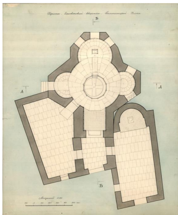
Рис. 6. План крещальни при Уваровской базилике Херсонеса (URL: http://orthodoxmoscow.ru/raskrytaya-tajna-oktagona/ )
