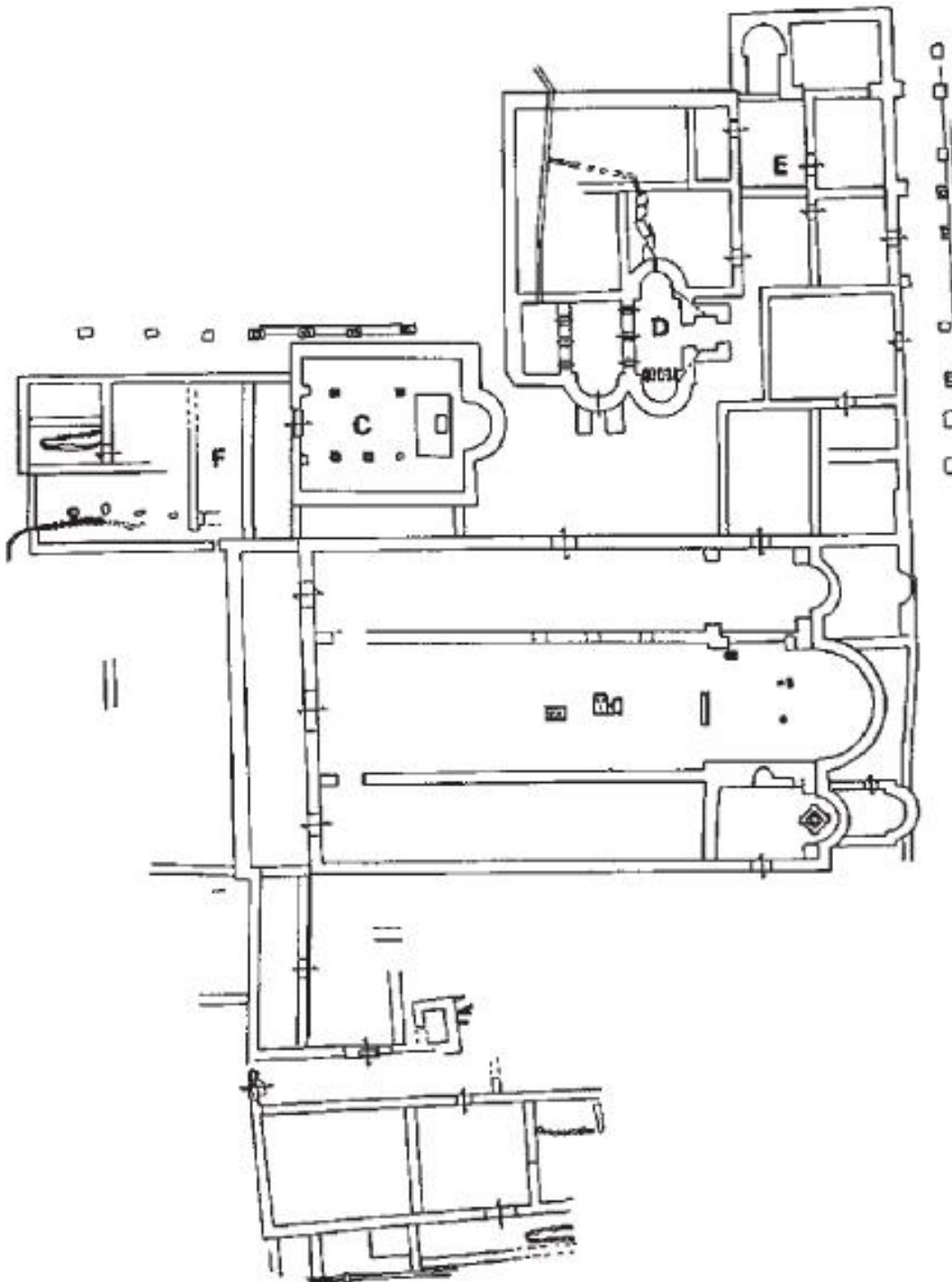
Рис. 8. План базилики в г. Нове (Болгария) (Виернаски А.В. 2005. A City of Christians: Novae in the 5 th and 6 th C AD. Archeologia Bulgarica IX, No 1. Sofia, 53–74)
